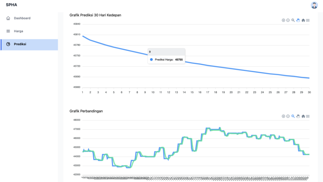
Gambar 15. Tampilan Prediksi Pengguna
