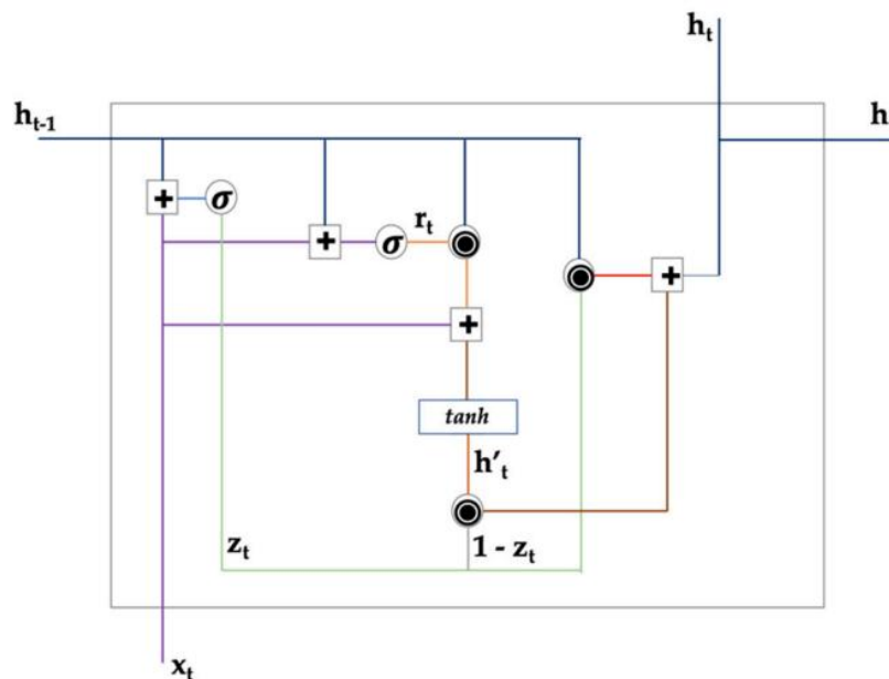
Gambar 2. Struktur GRU
